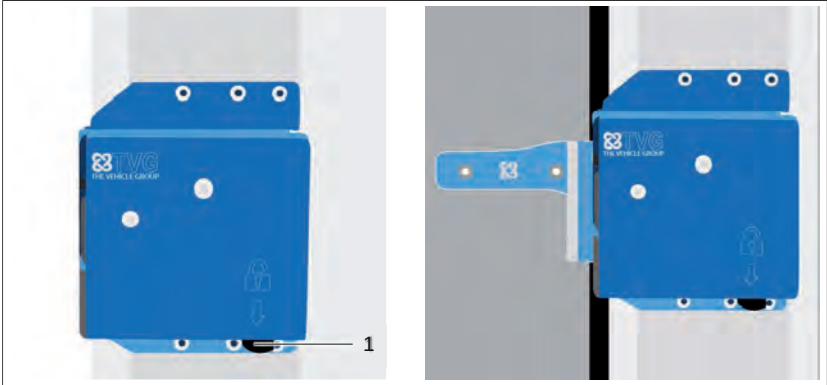
Illustration 11 : Système de verrouillage des portes du compartiment de chargement - marque TVG, vue (à gauche), état fermé (à droite)
