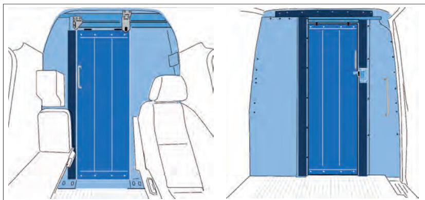
Abbildung 25 Trennwand mit Schiebetür, Ansicht Fahrerraum (links), Ansicht Laderaum (rechts)
