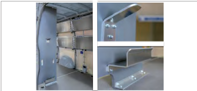
Abbildung 5: Paketkarrenhalter ohne Karre (links), Details (rechts)
