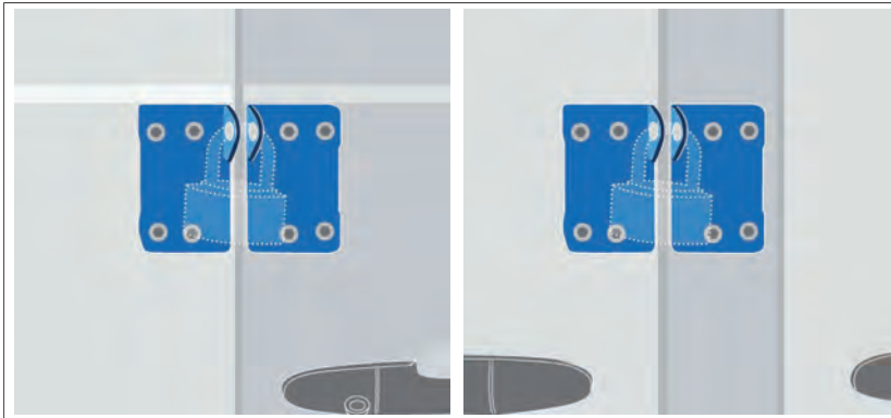
Abbildung 22: Beschläge für Vorhängeschloss, Hecktür (links), Laderaumschiebetür (rechts)
