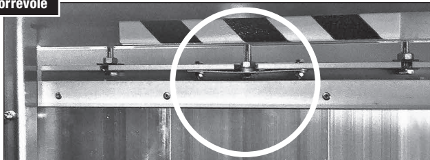
Figura 25 Parete divisoria con porta scorrevole, visione dal vano del conducente (sinistra), visione dal vano di carico (destra)
